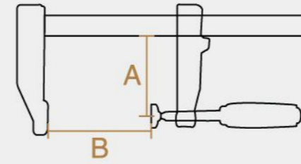
英式木工夹 Wood clamp, British type
